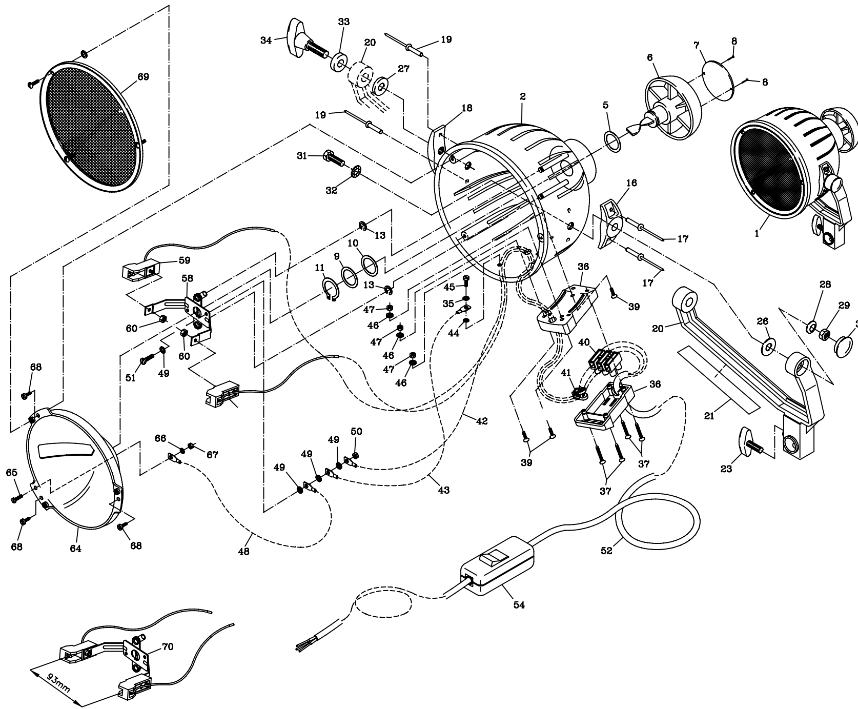
VARIBEAM Q1000 - ART. 1000 "ECO" ( PER LAMPADA LUNGA 93 mm )
