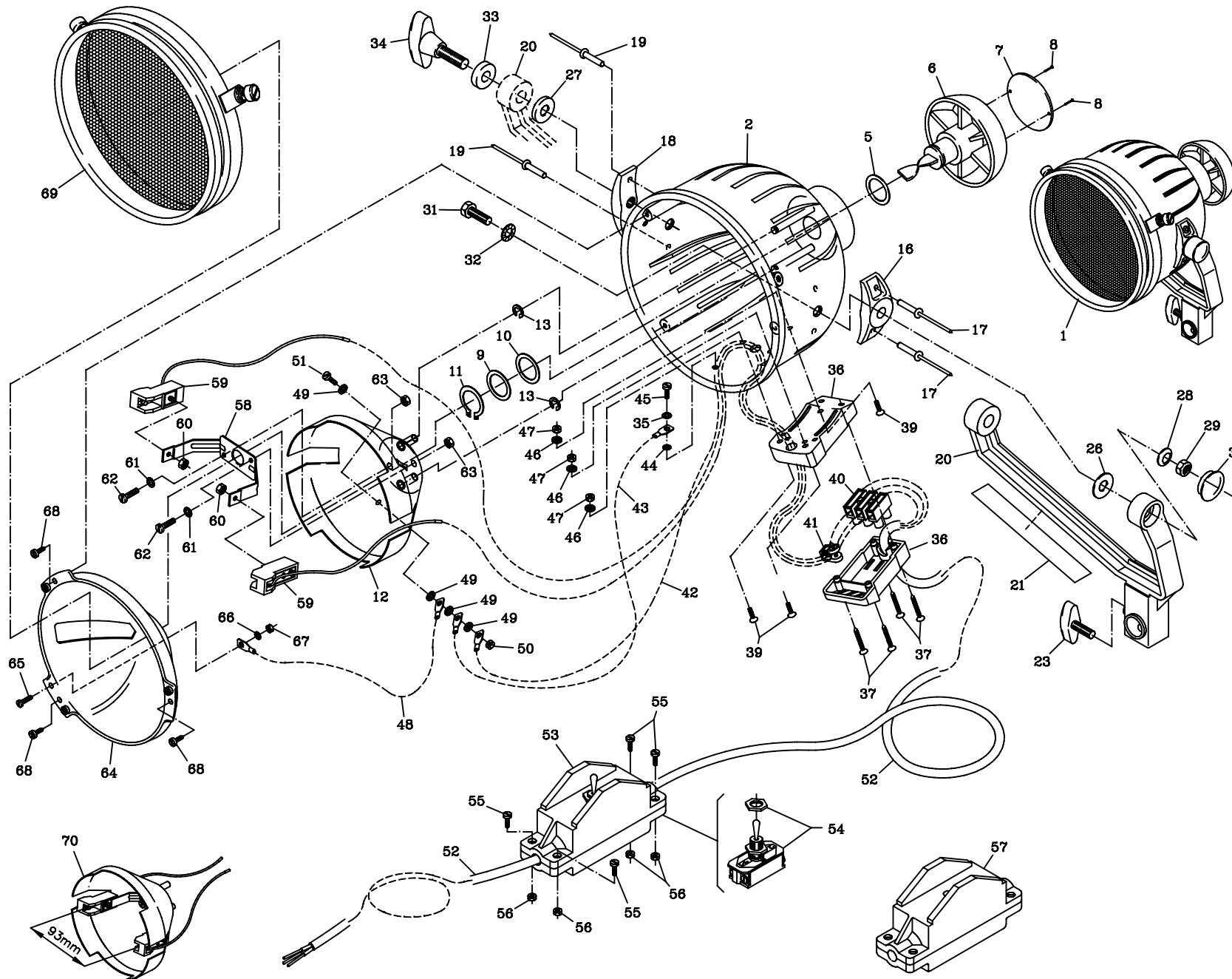
VARIBEAM Q1000 - ART. 1000 ( PER LAMPADA LUNGA 93 mm )
