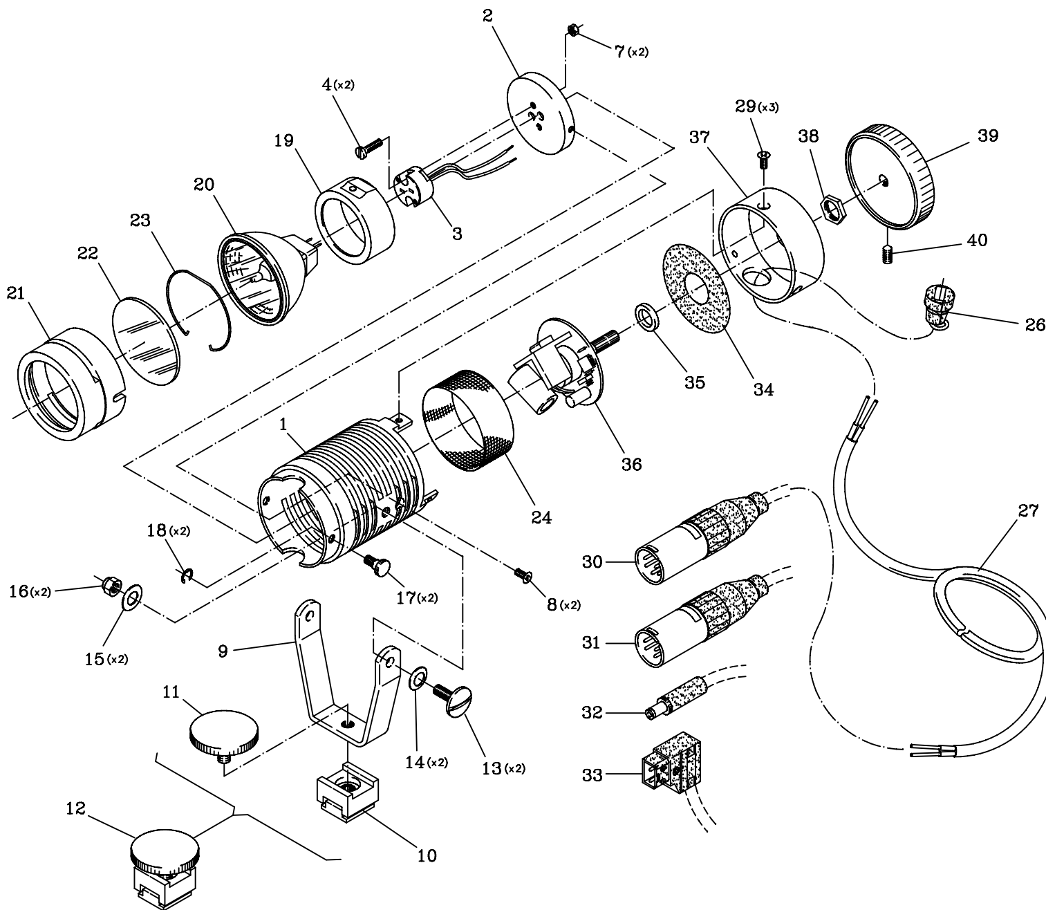
FARETTO "ALADINO" DIMMER - ART. 1910
