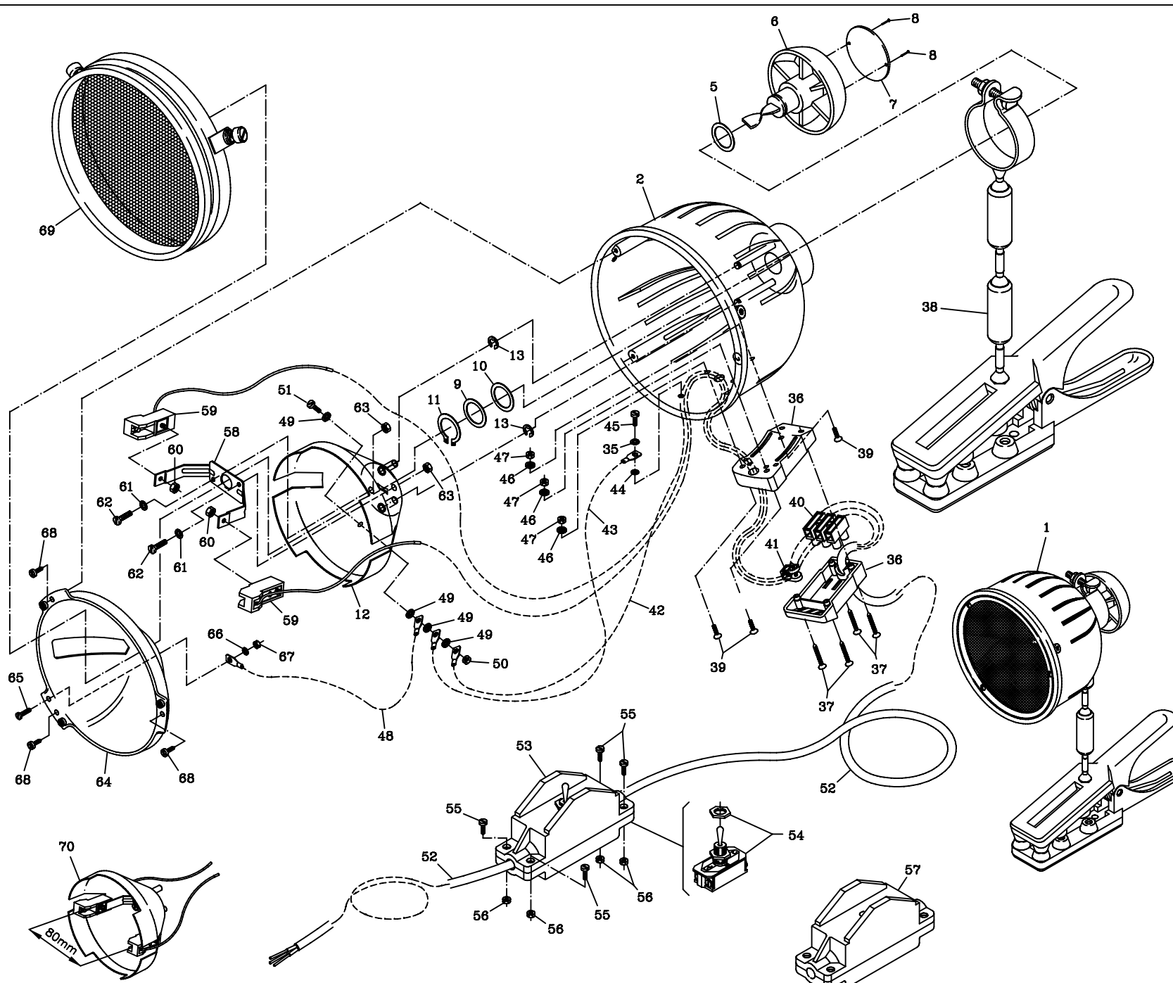
VARIBEAM Q800 - ART. 900 ( PER LAMPADA LUNGA 80 mm )
